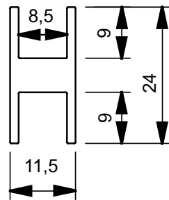
Einschuhprofil 606 310
