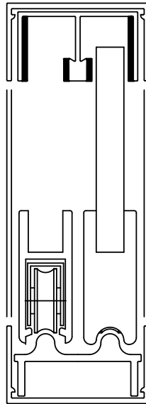
SUPRA-Rahmenbeschlag (Einschuhmaterial)
