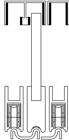
SUPRA-Dreibahnbeschlag
