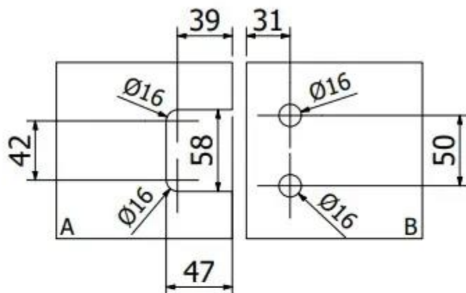
Výrez do skla s tesnením 8861
