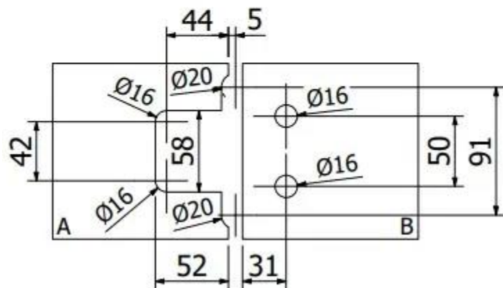
Výrez do skla bez tesnenia
